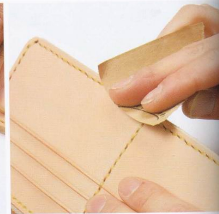
13 コ字型縫製完成之後，用削邊器削掉毛邊，再用砂紙讓皮革的高低差變得均勻。毛邊的高度有某種程度的一致之後，用手指塗上CMC，並用乾淨的布打磨。
