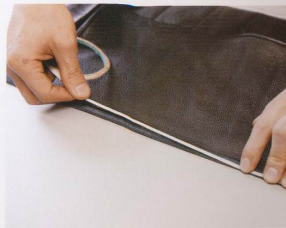
26 在距離袋身邊緣10mm寬的地方貼上袋蓋，並在反折部分貼上膠帶。
