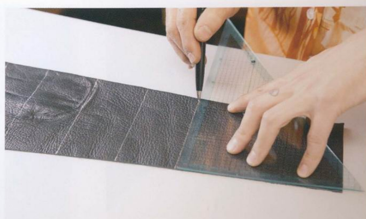
15 在工具插袋(光滑面)上，依序從左邊開始畫出40mm寬、50mm寬、50mm寬、60mm寬、60mm寬、60mm寬、60mm寬、100mm寬的直線。就算要改變寬度也沒關係。
