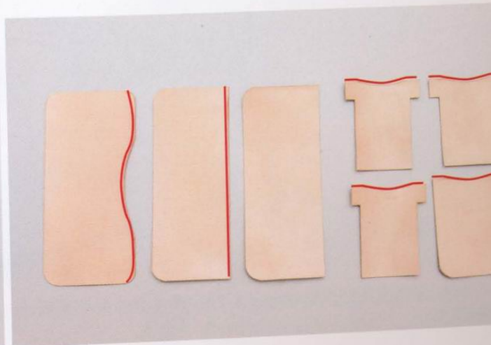
3 削掉邊緣部分的毛邊用含水的廢布料擦拭並塗上床面處理劑。在這裡使用的是背面處理劑。將多餘的背面處理劑擦掉之後，用乾燥的菜瓜布和帆布打磨。乾燥的菜瓜布多半在超市或生活用品賣場的浴室用品專櫃等地方販售。
