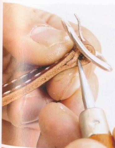
29 用錐子等工具將線結壓進裡面看不見的地方。為了不要讓線結鬆開，所以要塗上接合劑來固定。
