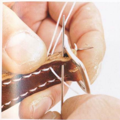
27 縫製的最後，將兩支針貼在一起，從兩片皮革中間穿出來。和尖端那邊用相同的方法固定雖然也沒問題，但是像這樣做的話則可以隱藏線結的痕跡。
