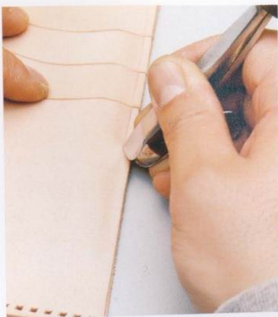
8 在剝掉背皮的狀態下，在鈔票夾口的附近畫出導引線，並用菱斬鑽出縫線孔。在這裡要將暫時固定的內袋D剝掉。
