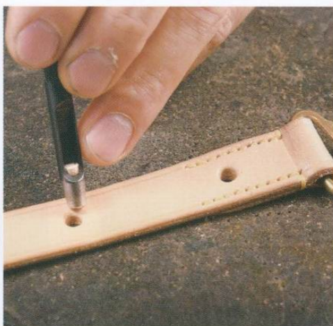
19 在這裡要使用彈簧釦。將彈簧釦公的部分從袋身插入，壓在皮帶上並做出記號，然後再用丸斬在做記號的位置上鑽孔。
