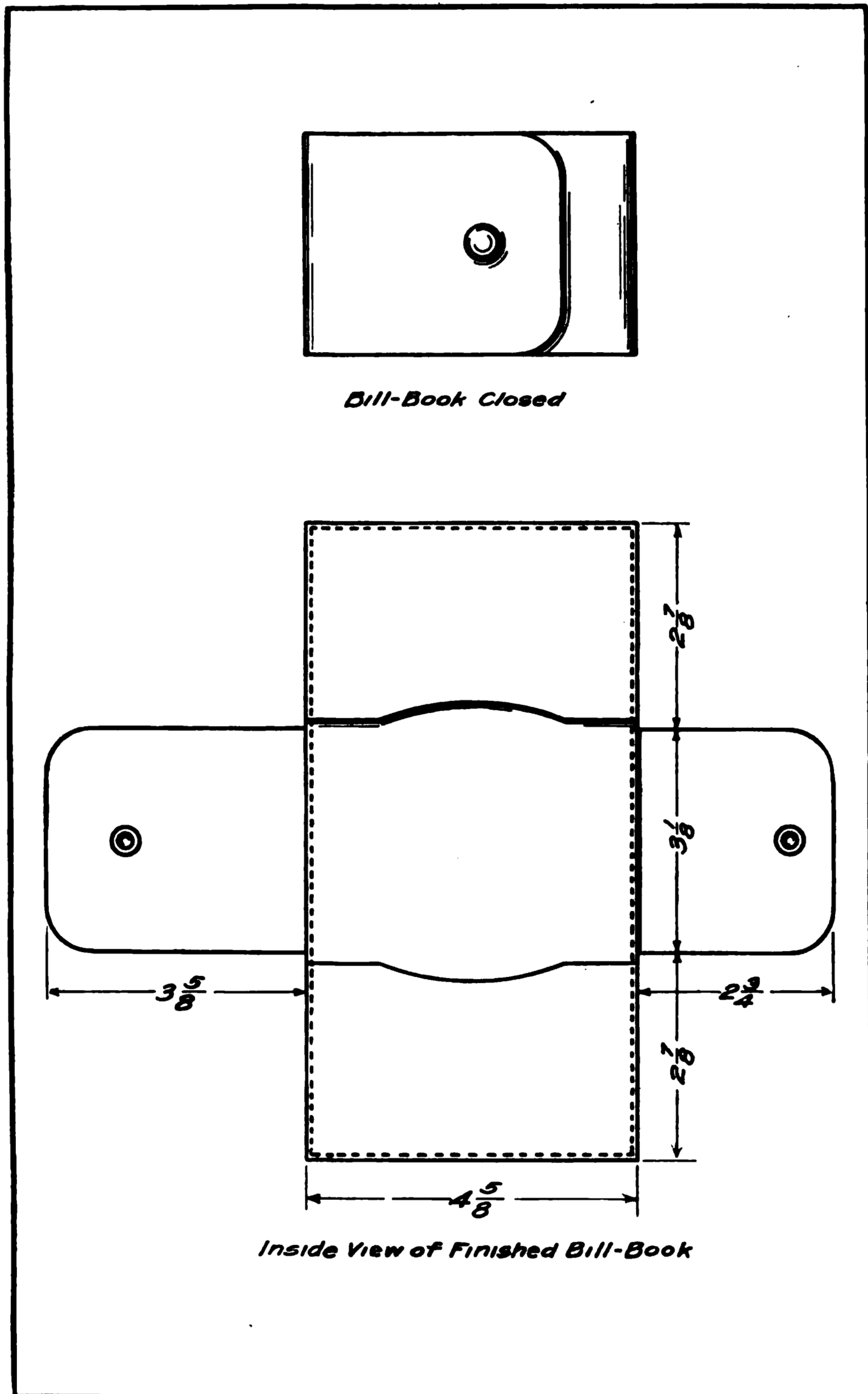
Fig. 21. Bill-Book.
