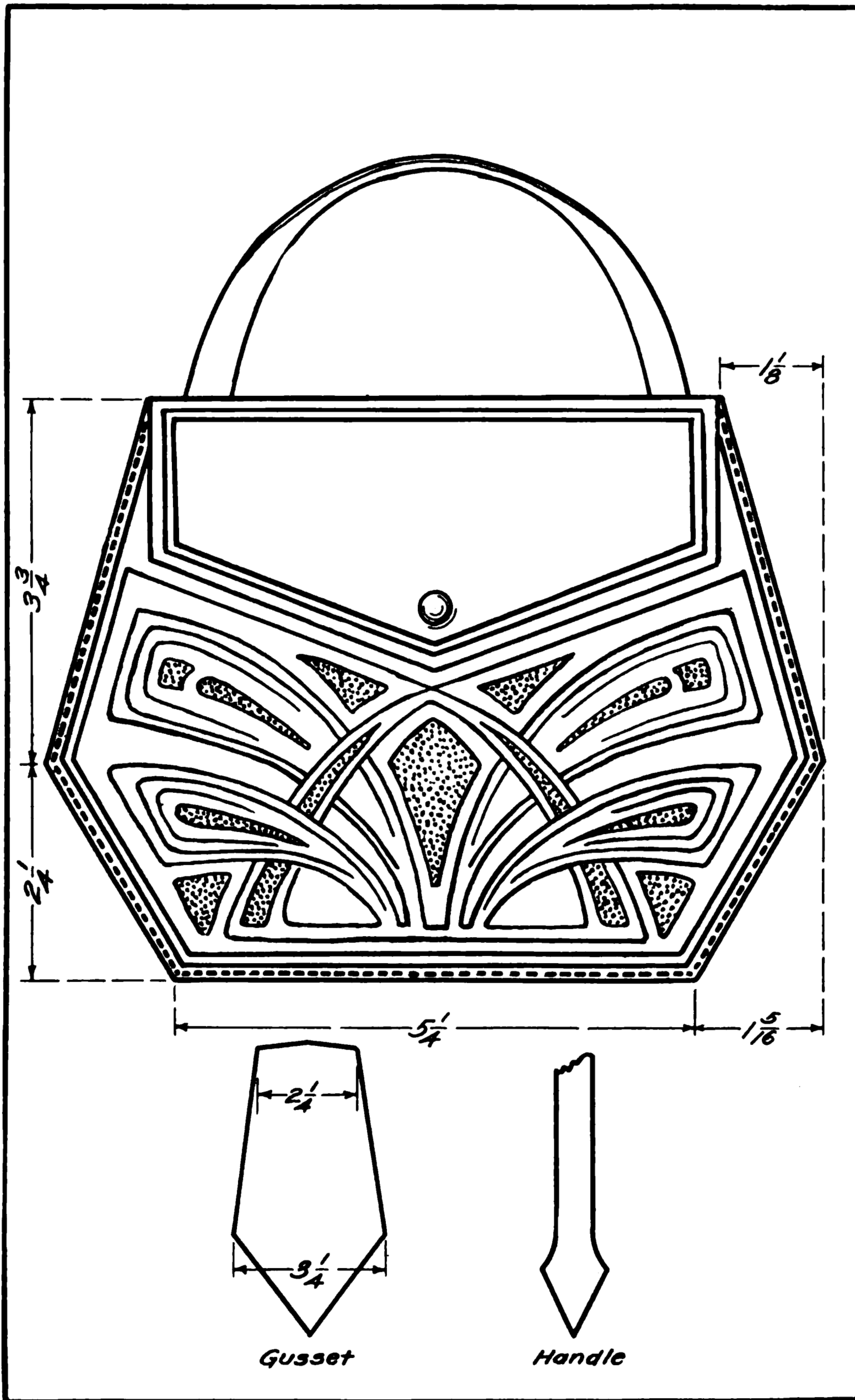
Fig. 32. Hand-Bag.
