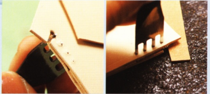
8 從距離邊緣 7mm 之處開始以菱斬鑿出縫孔。只有第一支刀刃不要刺到邊皮。下面墊張小塊皮革，有助作業進行。
