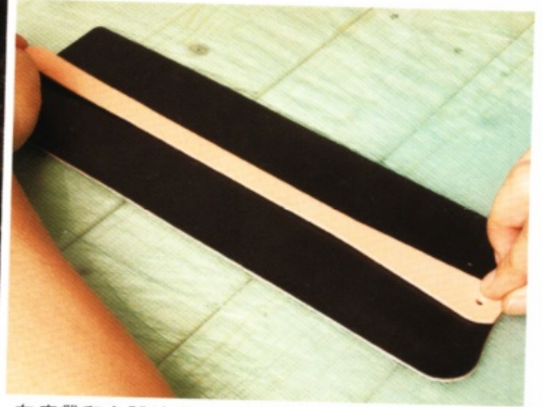
6 用圓斬鑽出安裝原子釦的孔位。在皮帶和主體塗上橡皮黏膠，再將皮帶輕輕置於主體。
