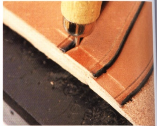
4 在以菱斬壓出印記前，用鐵筆在皮革重疊的部分做記號。
