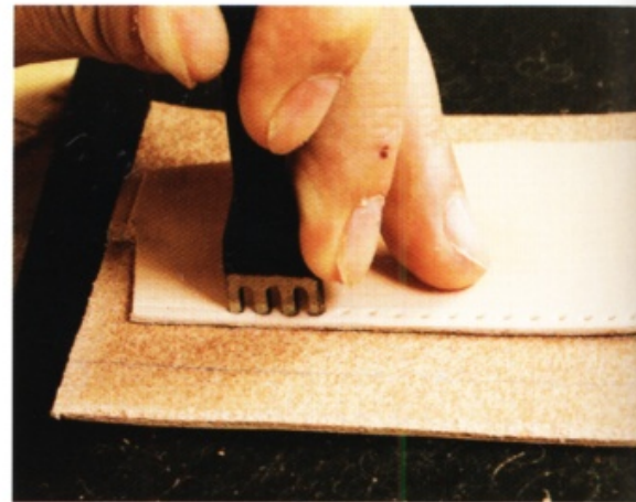
10 用菱斬鑿出縫線孔。鑿出所有的縫線孔後，接下來準備縫合。
