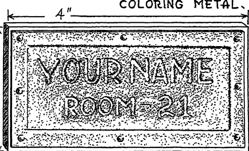
Fig. 2. DOOR PLATE.
