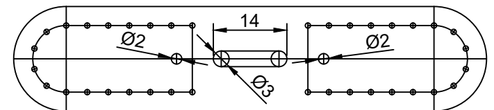
Держатель полукольца
