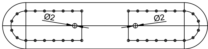
Держатель полукольца
