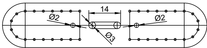
Держатель полукольца
