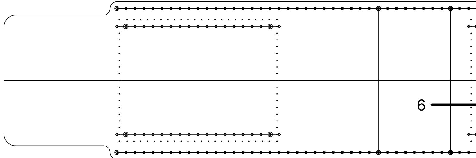
Держатель пряжки(запряжник)
